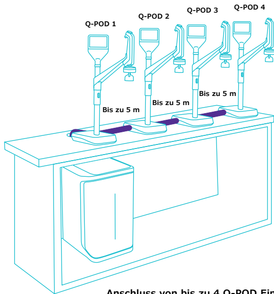
Anschluss von bis zu 4 Q-POD Einheiten
