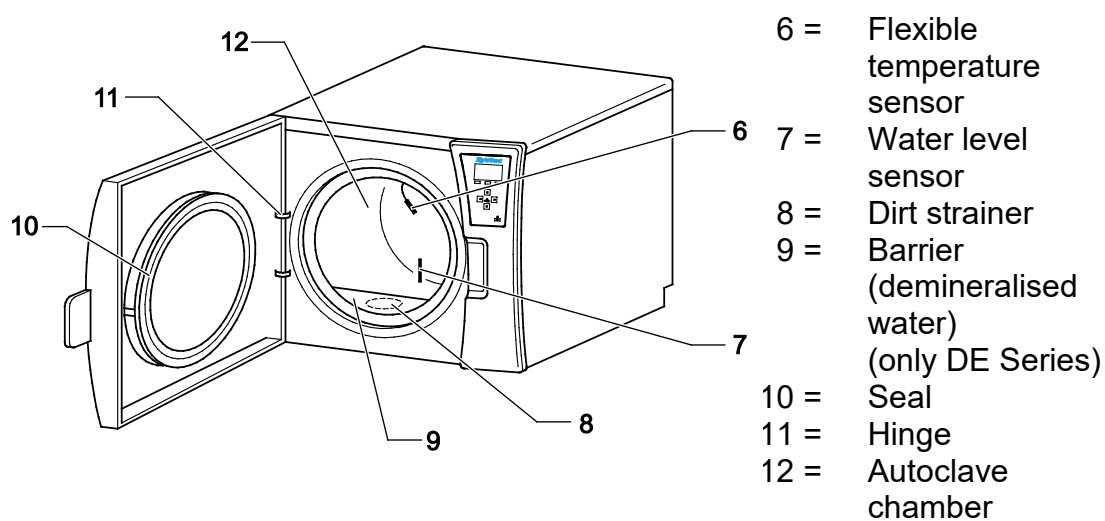
Fig. 2: Systec DX/DE Series; door open
