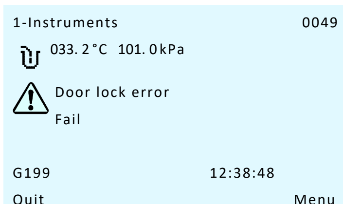
Fig. 17: Display message Door lock error if the door is not locked correctly
